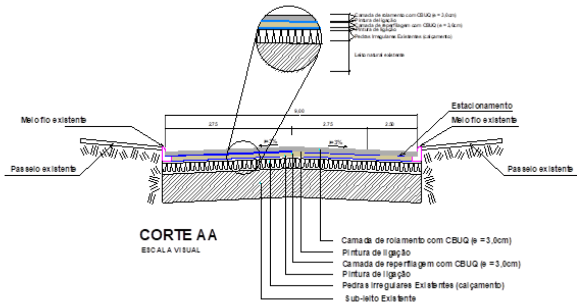
Detalhe 01 – Execução de pavimentação sobre calçamento
