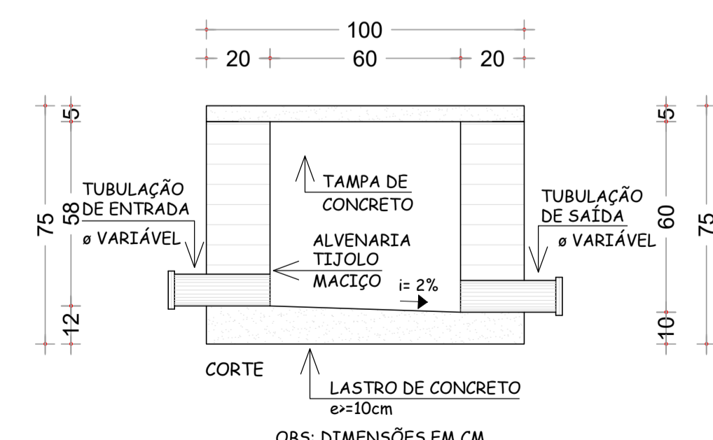
CAIXA DE INSPEÇÃO ESCALA: 1:20
