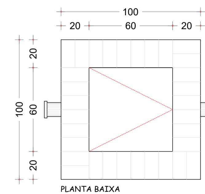
PLANTA BAIXA
