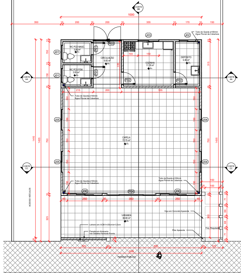
IMPLANTAÇÃO - PLANTA LAYOUT 1 : 75
