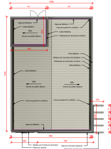
IMPLANTAÇÃO - PLANTA DE COBERTURA 1 : 75
