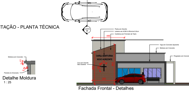
Fachada Frontal - Detalhes 1 : 75
