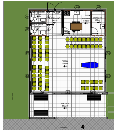
IMPLANTAÇÃO - PLANTA LAYOUT 1 : 75
