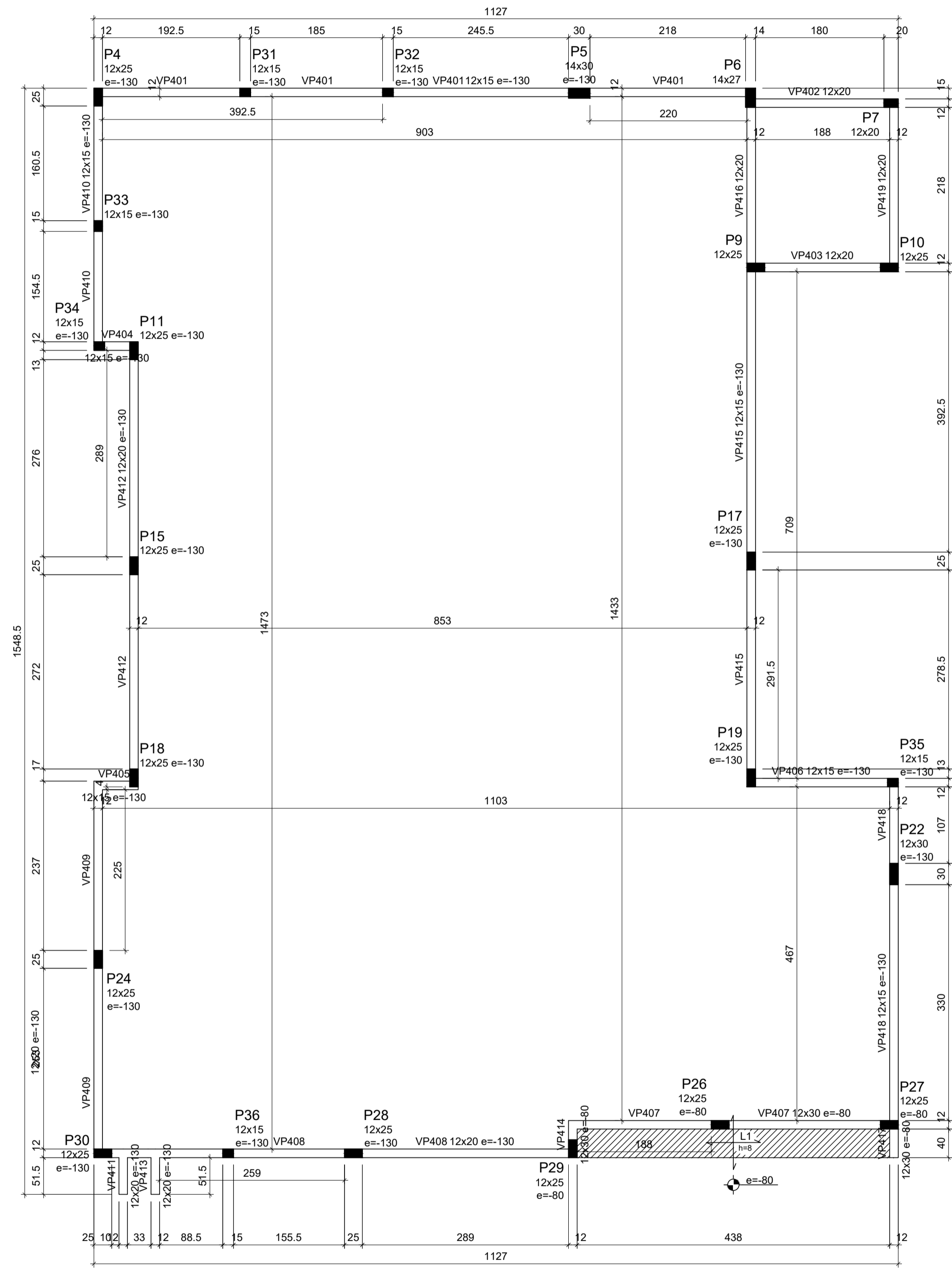
Forma do pavimento Volume (Nível 870) escala 1:50
